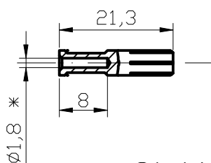
Styki wielowtyku
